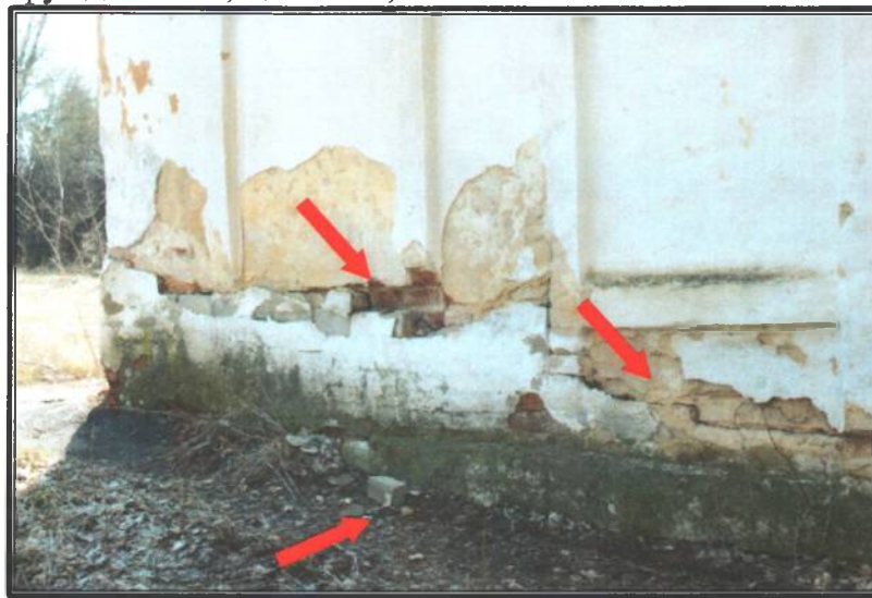
Фото 1. Объект культурного наследия регионального значения «Усадьба Нечаевых». Воронежская обл., Семилукский р-н, с. Терновое, ул. Терновская, 2. Разрушение кирпичной кладки в уровне цоколя. Отсутствие отмостки по периметру. Фото Попова А.А., март 2016 года
