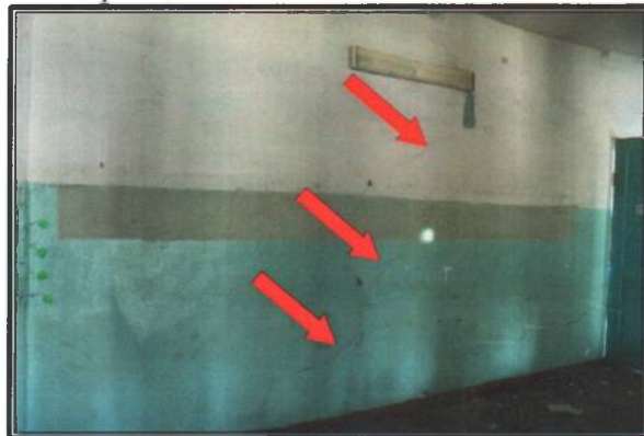
Фото 3. Объект культурного наследия регионального значения «Усадьба Нечаевых». Воронежская обл., Семилукский р-н, с. Терновое, ул. Терновская, 2. Вертикальные сквозные трещины в несущей стене. Фото Попова А.А., март 2016 года
